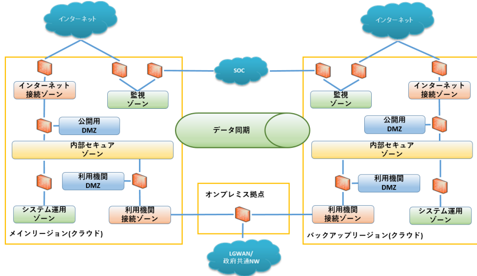
(1) システム概要図
